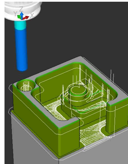
上图：用ACC功能铣削的零件 下图：未用ACC功能铣削的零件
